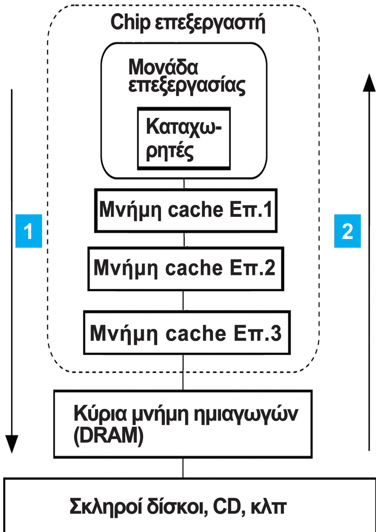
Σχήμα 1.4. Ιεραρχία μνήμης
